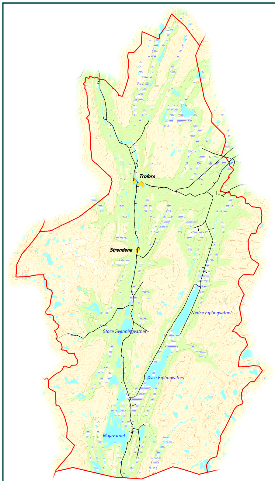
Figur. 4.1: Grane kommune med høyspent distribusjonsnett
