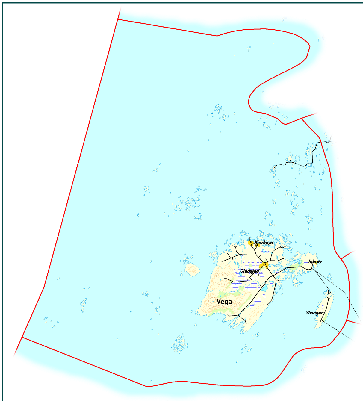
Figur. 4.1: Vega kommune med høyspent distribusjonsnett
